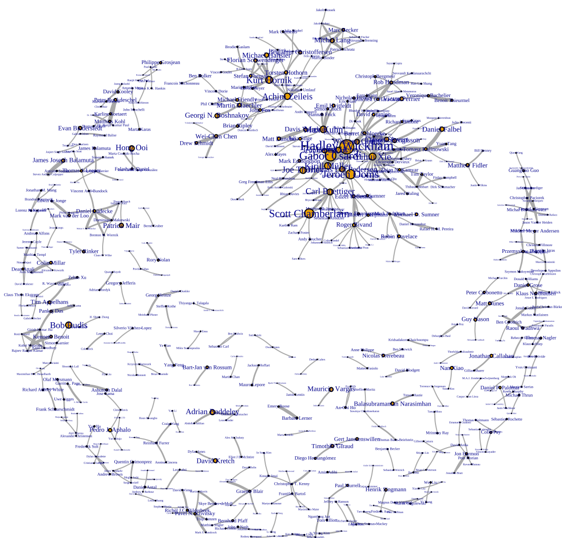
图 18.6: 开发者的协作关系网络
