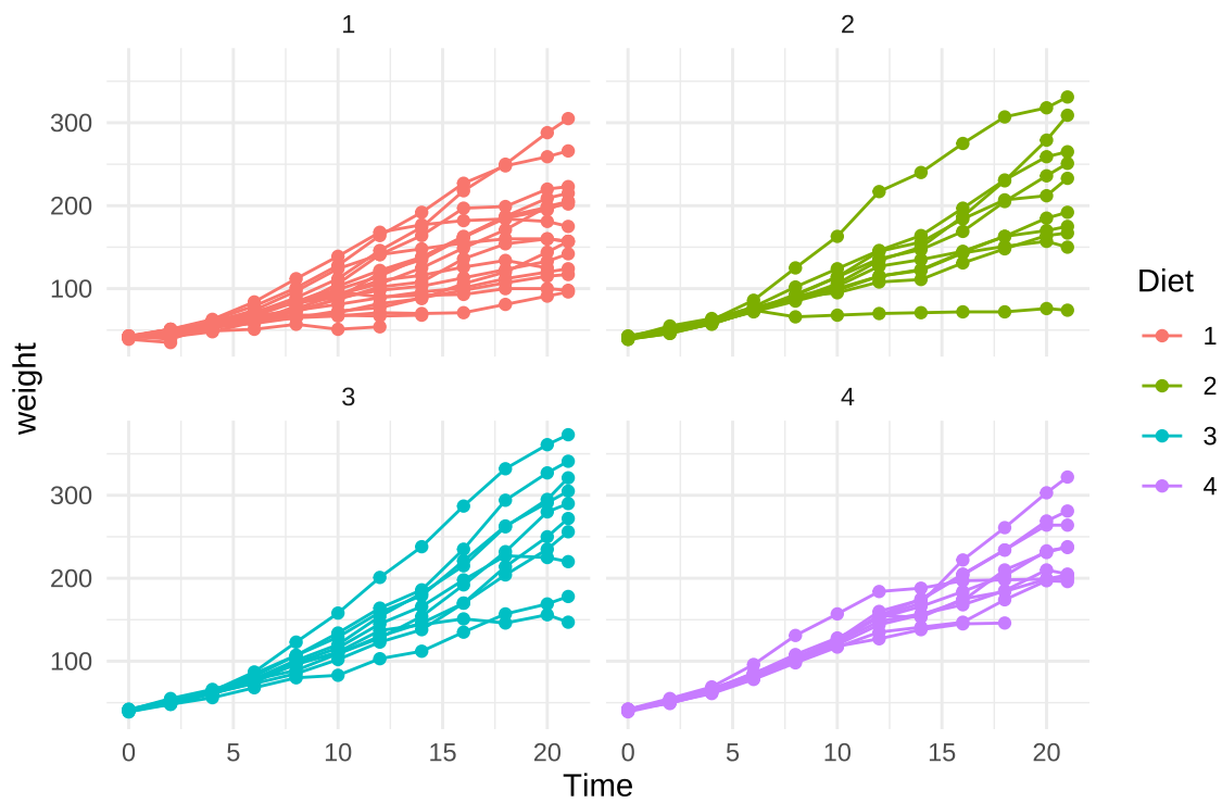
图 14.13: 不同喂食方式对小鸡的影响 (续)
