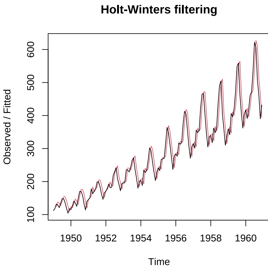
图 21.11: holt 指数平滑模型
