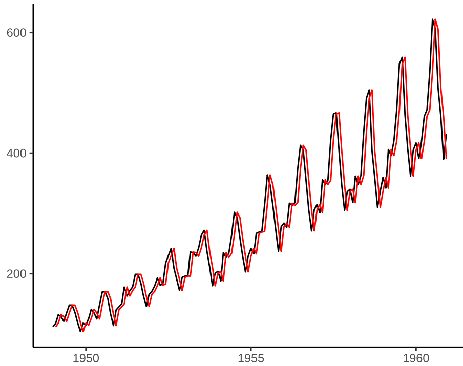
图 21.9: 简单指数平滑模型
