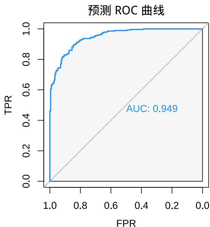
图 22.5: ROC 曲线
