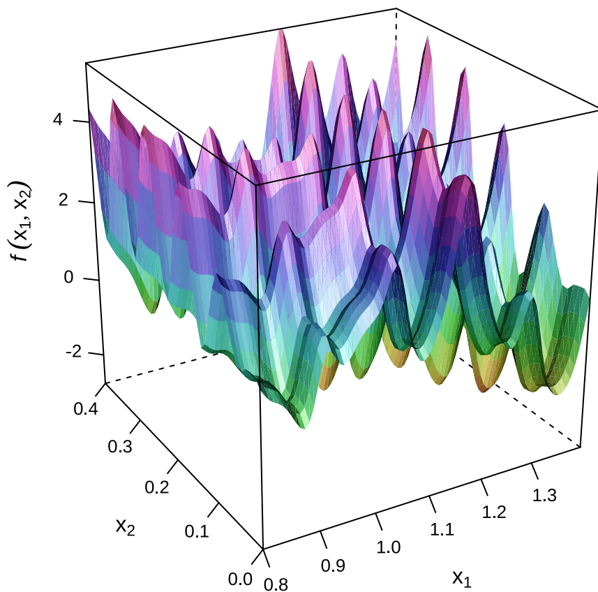
图 23.10: 目标函数的曲面图
