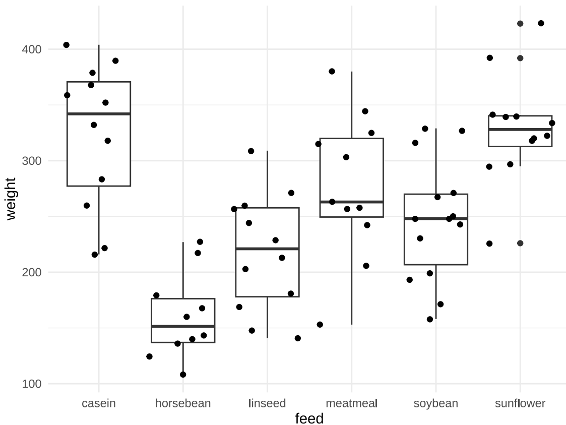
图 14.12: 不同喂食方式对小鸡的影响
