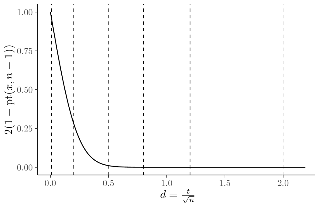
图 17.1: t 检验的功效
