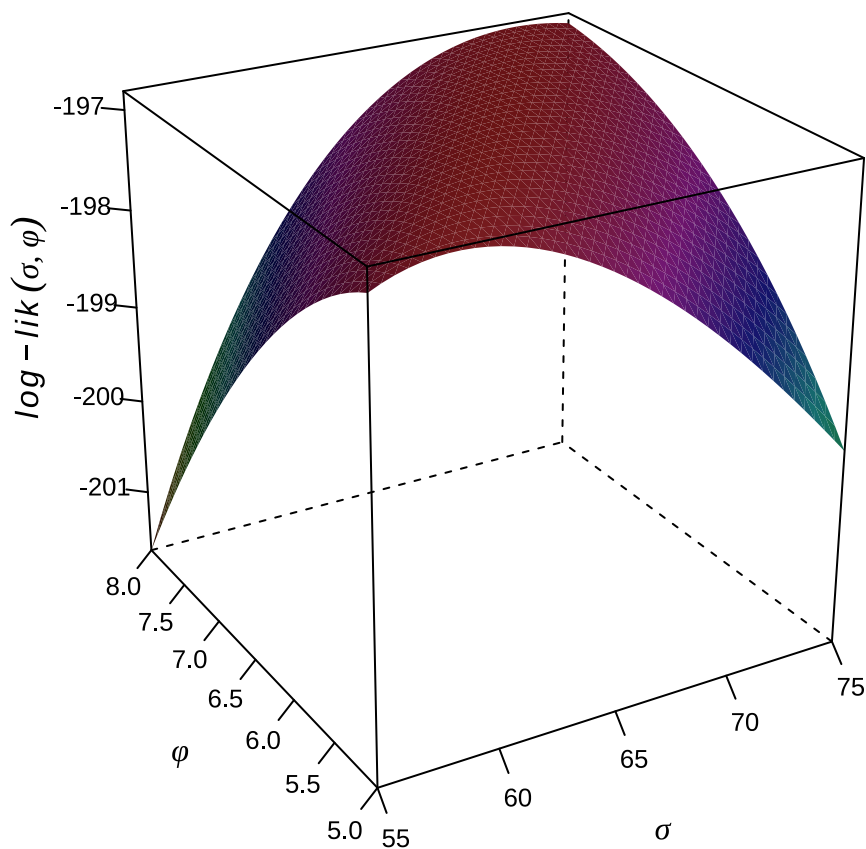
图 24.3: 对数似然函数的曲面图
