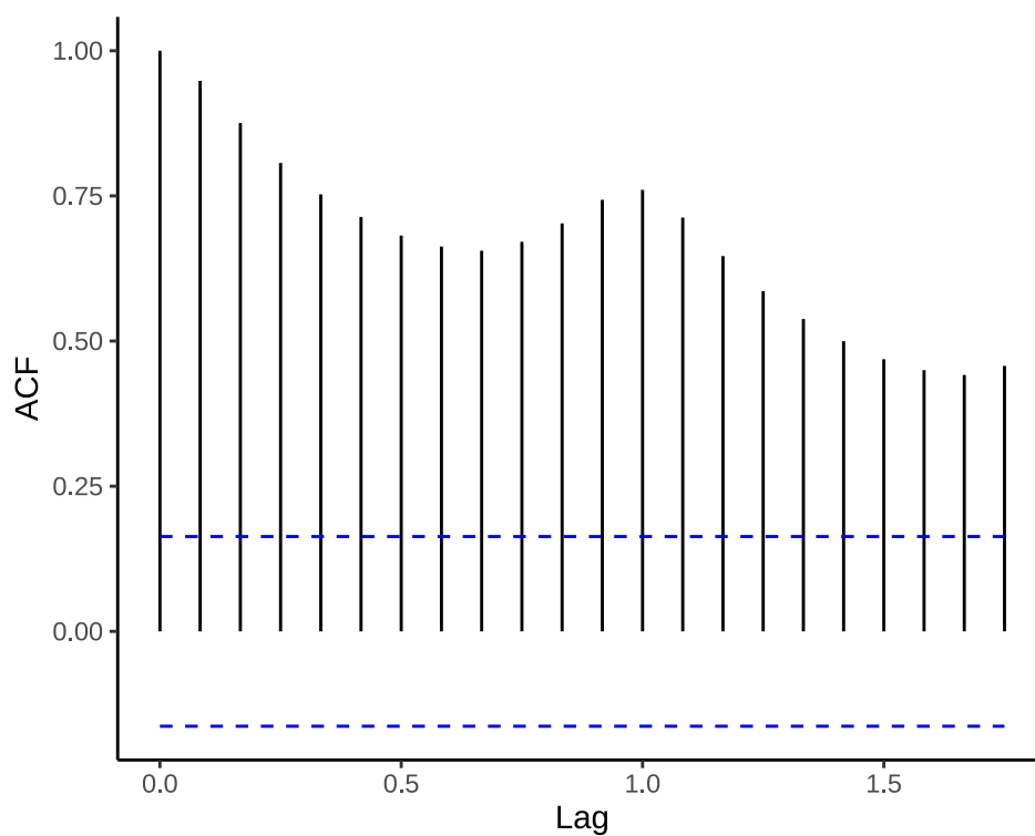
图 21.7: 乘客数量自相关图
