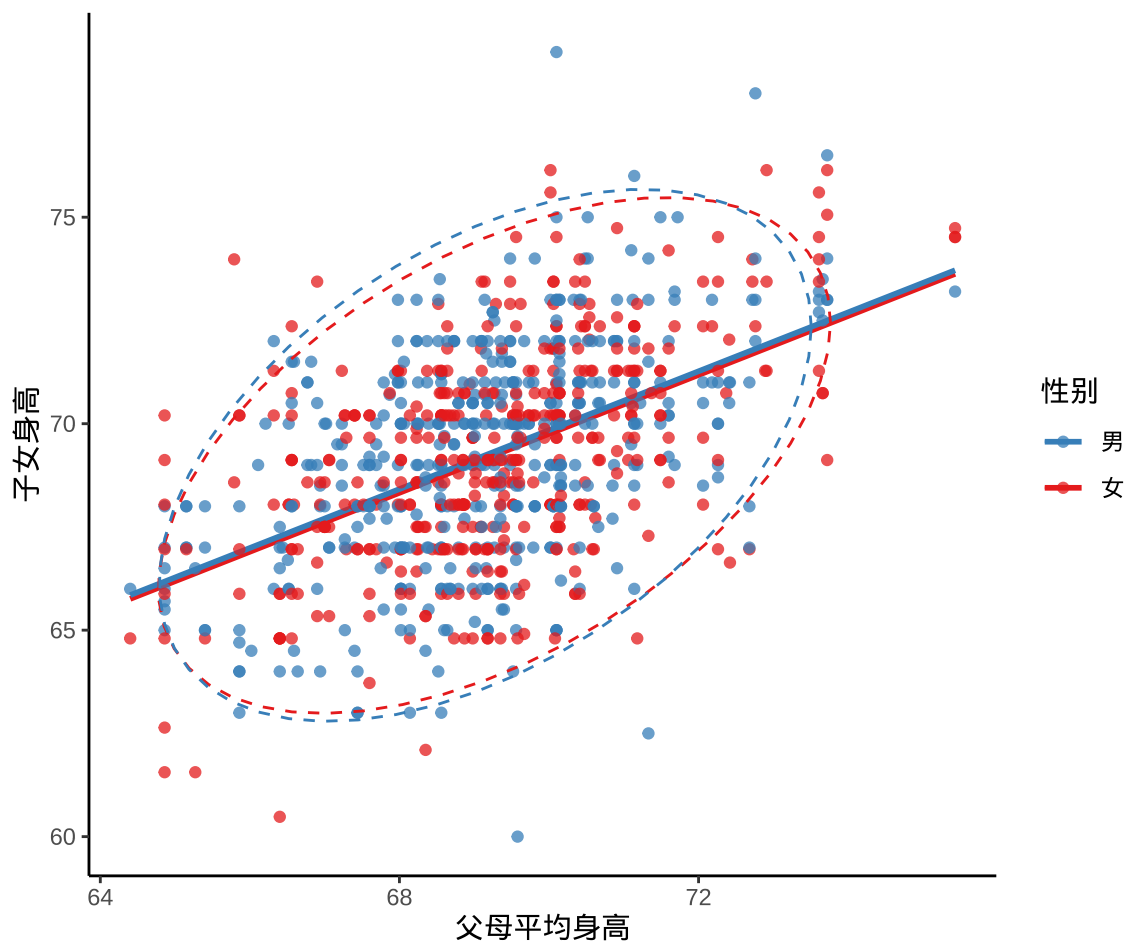
图 15.2: 子代身高与亲代身高的关系
