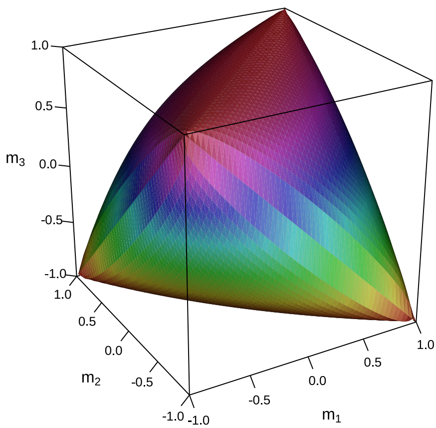
图 23.4: 锥
