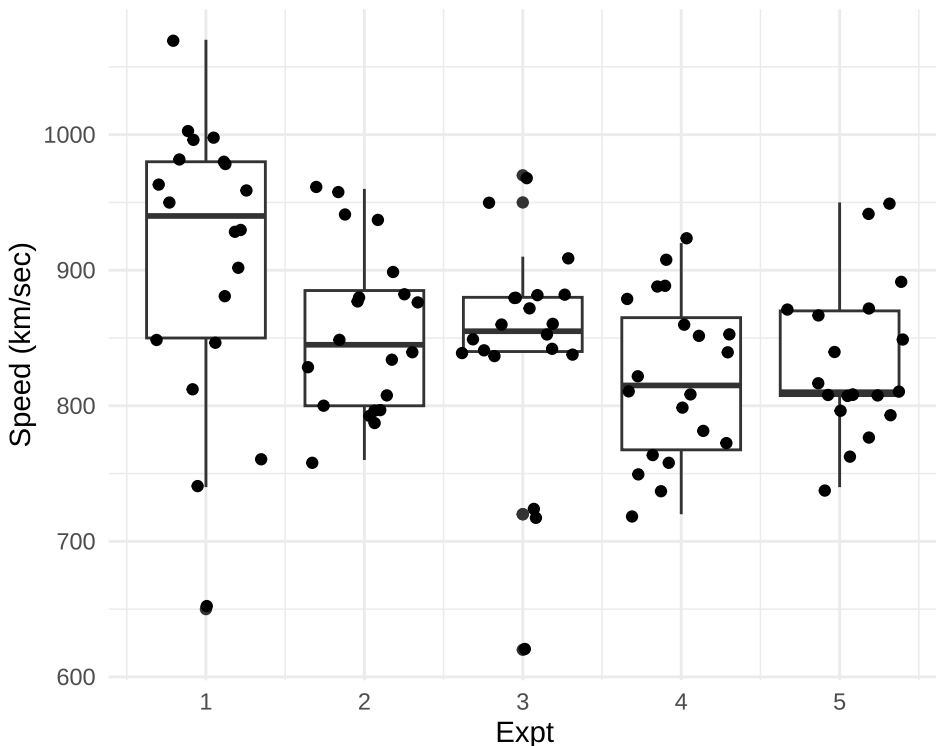
图 14.8: 1879 年迈克尔逊光速实验数据
