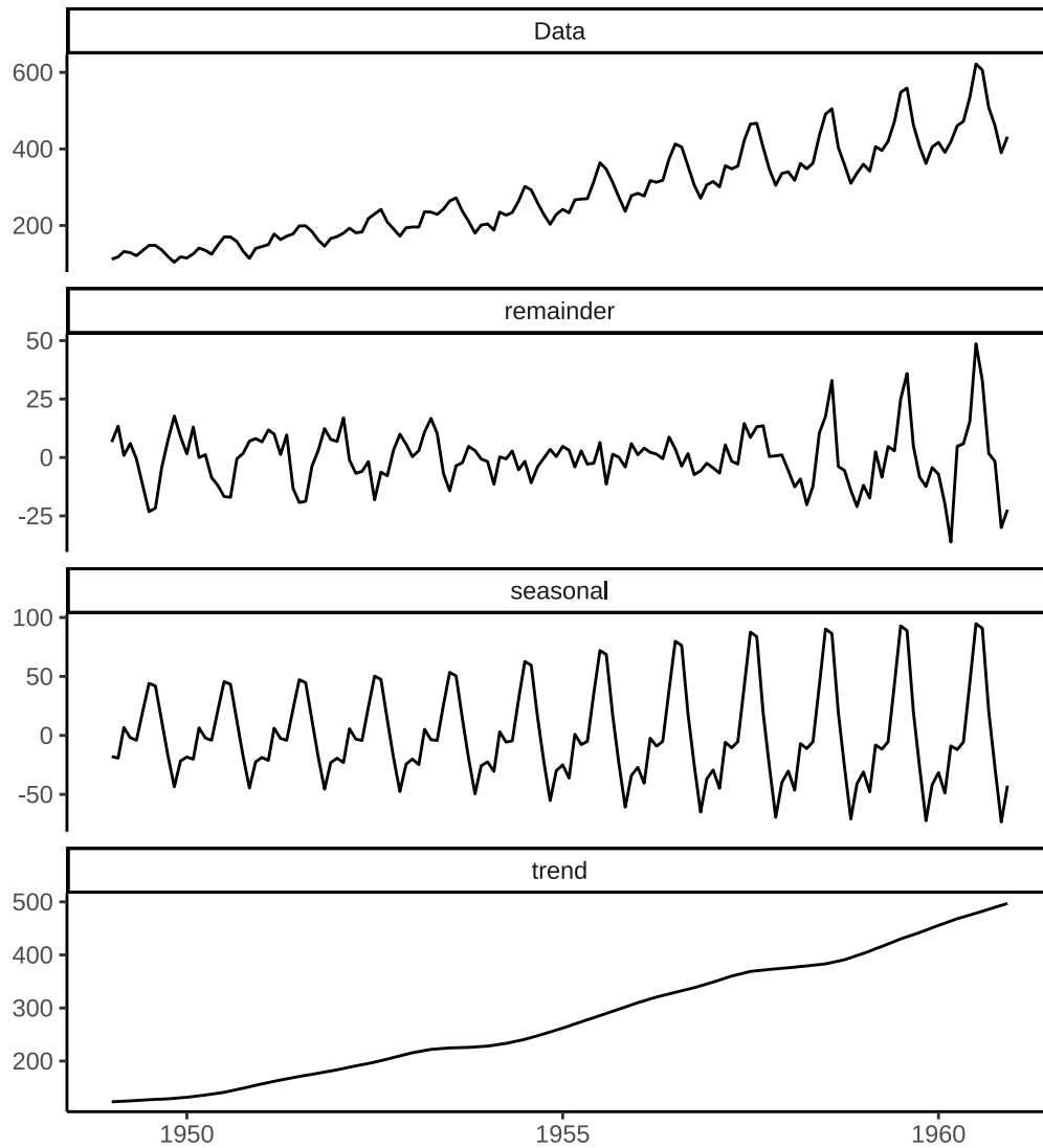
图 21.16: 变化趋势的分解
