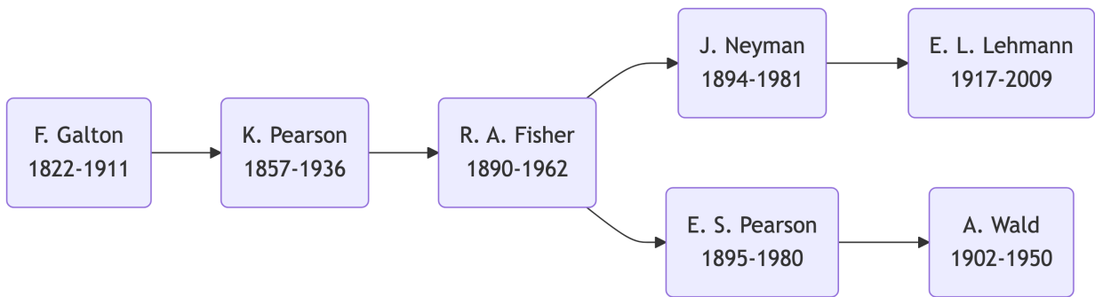
图 14.9: 最重要的统计学家及其学术传承关系
