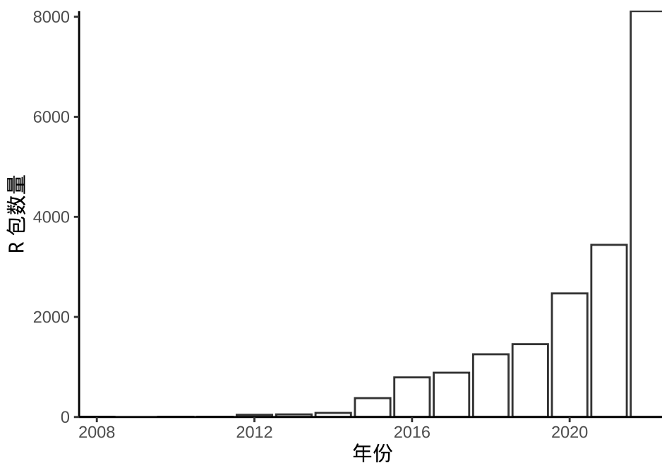
图 18.1: CRAN 上 R 包的更新情况
