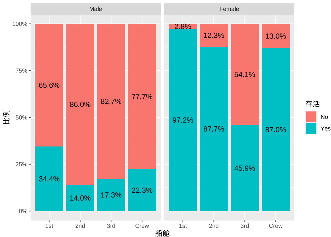
图 16.1: 百分比堆积柱形图展示多维分类数据
