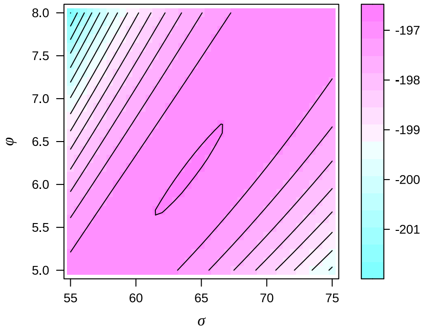
图 24.4: 对数似然函数的等高线图
