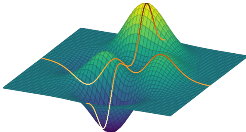
图 11.5: Peaks 函数图像
