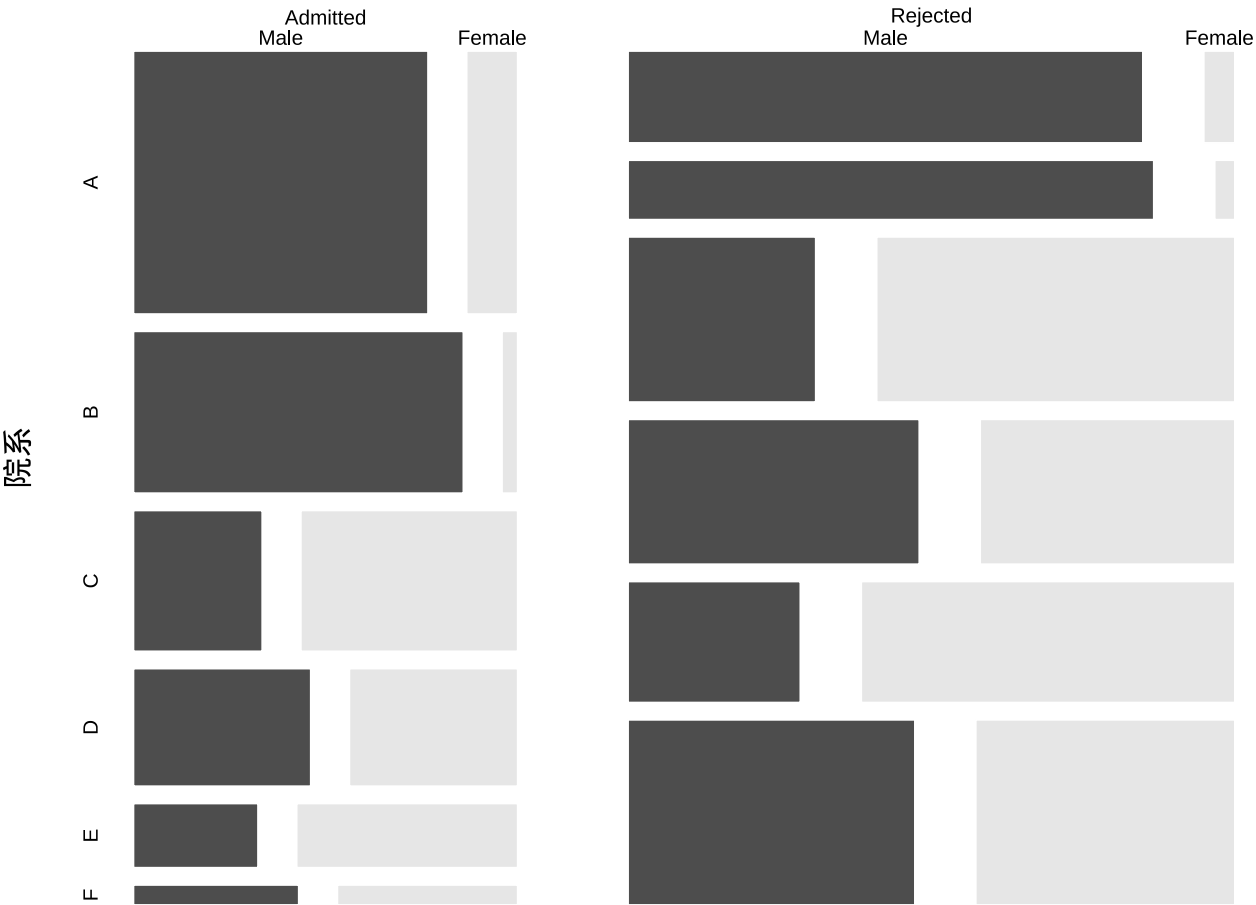
图 16.5: 加州伯克利分校院系录取情况
