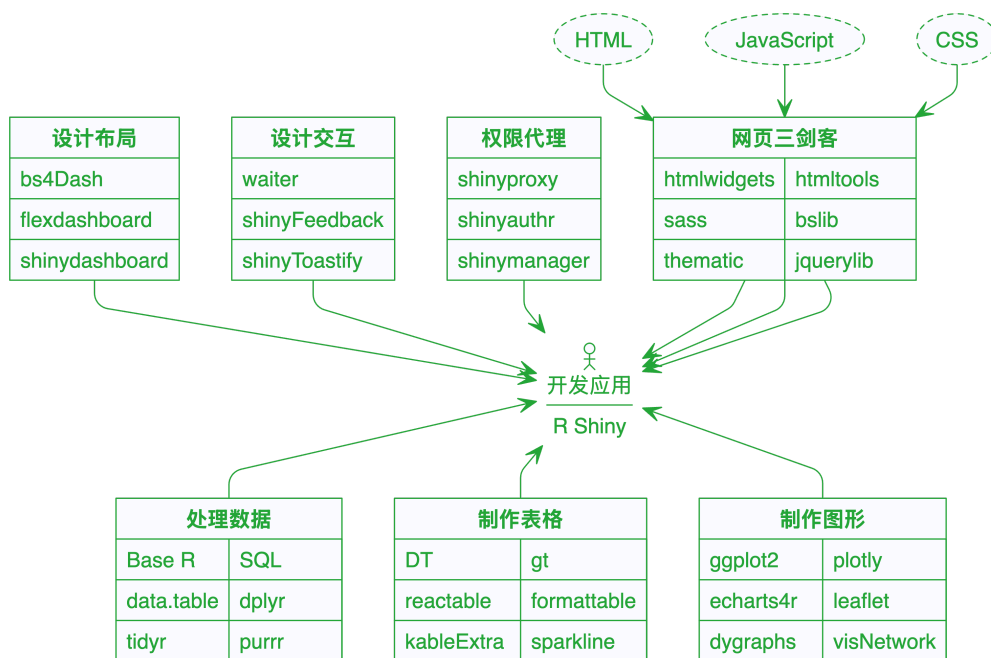
图 9.1: Shiny 生态系统
