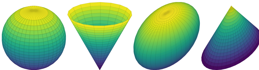
图 23.3: 常见的三维凸锥
