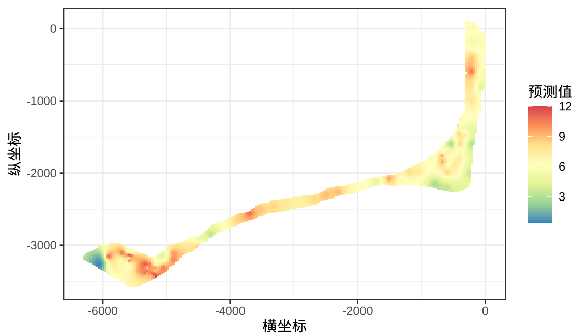
(a) 核辐射强度的预测值
