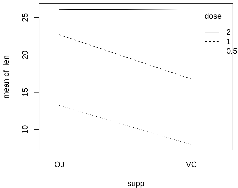
图 14.10: OJ 和 VC 的交互作用
