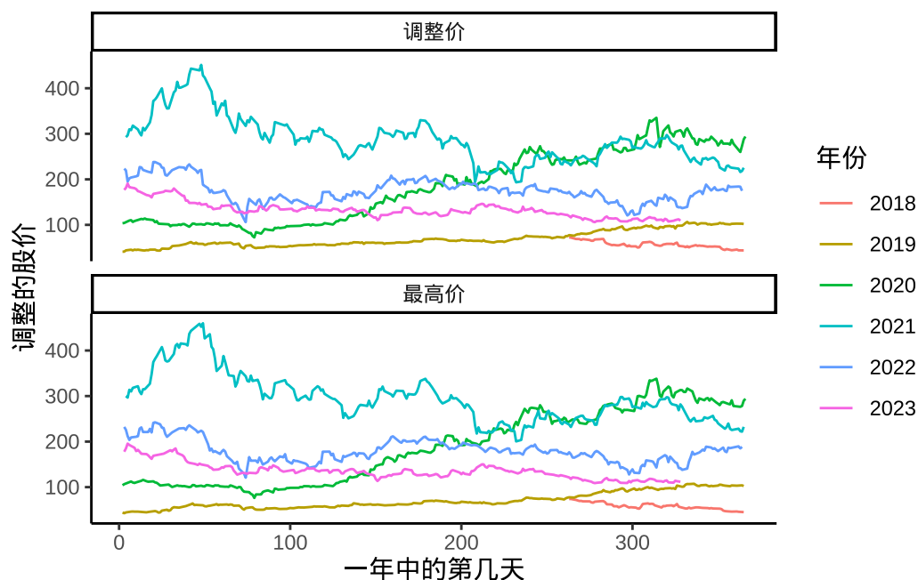
图 21.2: 美团调整的股价逐年走势
