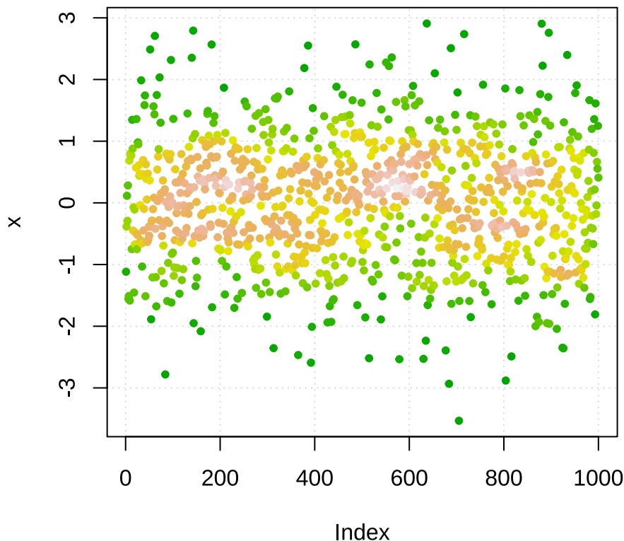
图 13.1: 一维正态分布
