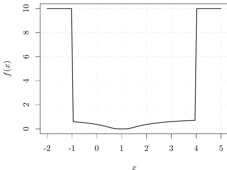
图 23.5: 一维函数图像
