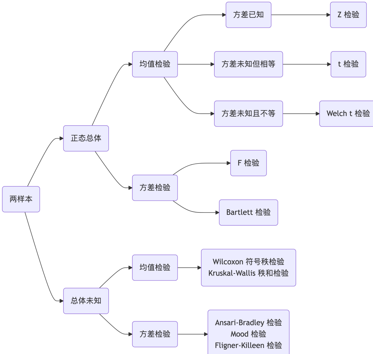
图 14.2: 两样本检验
