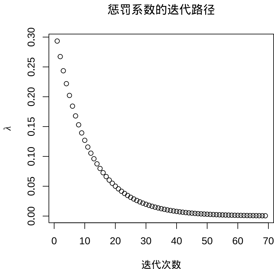
图 22.4: 惩罚系数的迭代路径
