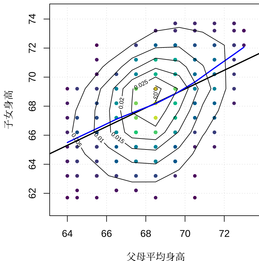
图 15.3: 二维核密度估计与二元正态分布
