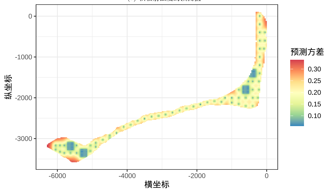
(b) 核辐射强度的预测方差
