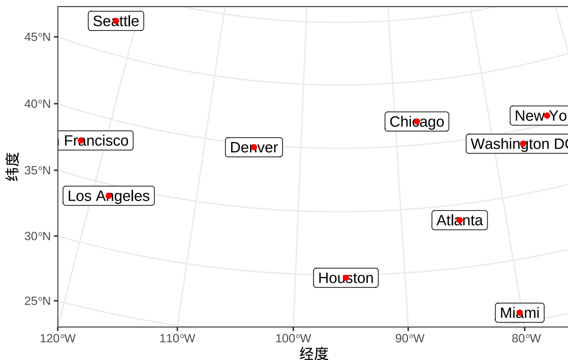
图 24.1: 10 个城市的分布图
