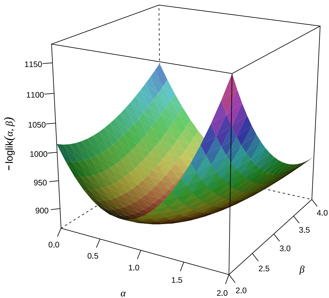
图 22.2: 二维情形下的逻辑回归模型的负对数似然函数曲面
