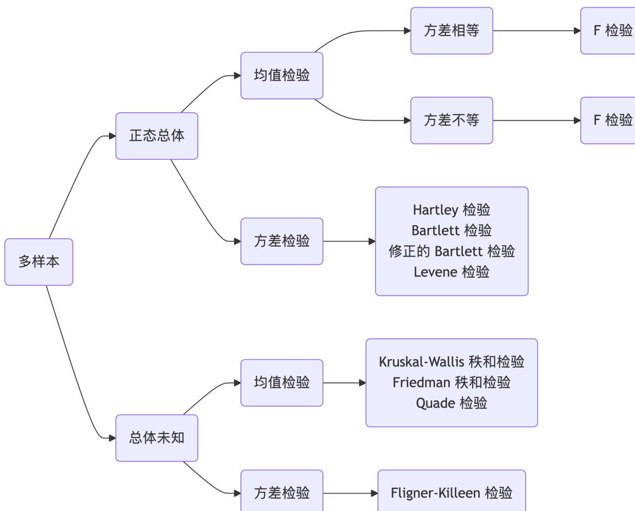
图 14.6: 多样本检验
