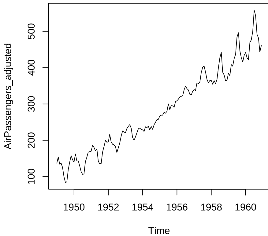
图 21.15: 季节性调整
