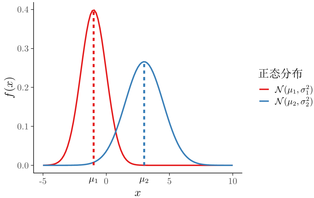
图 14.3: 两样本均值之差的检验
