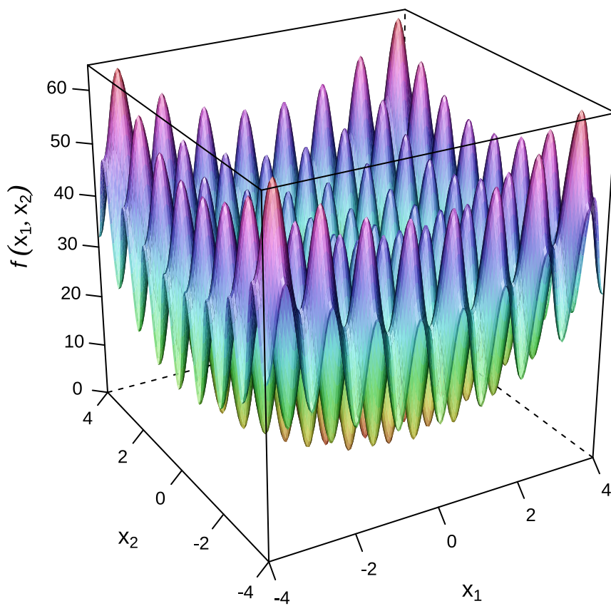
图 23.7: 二维 Rastrigin 函数图像
