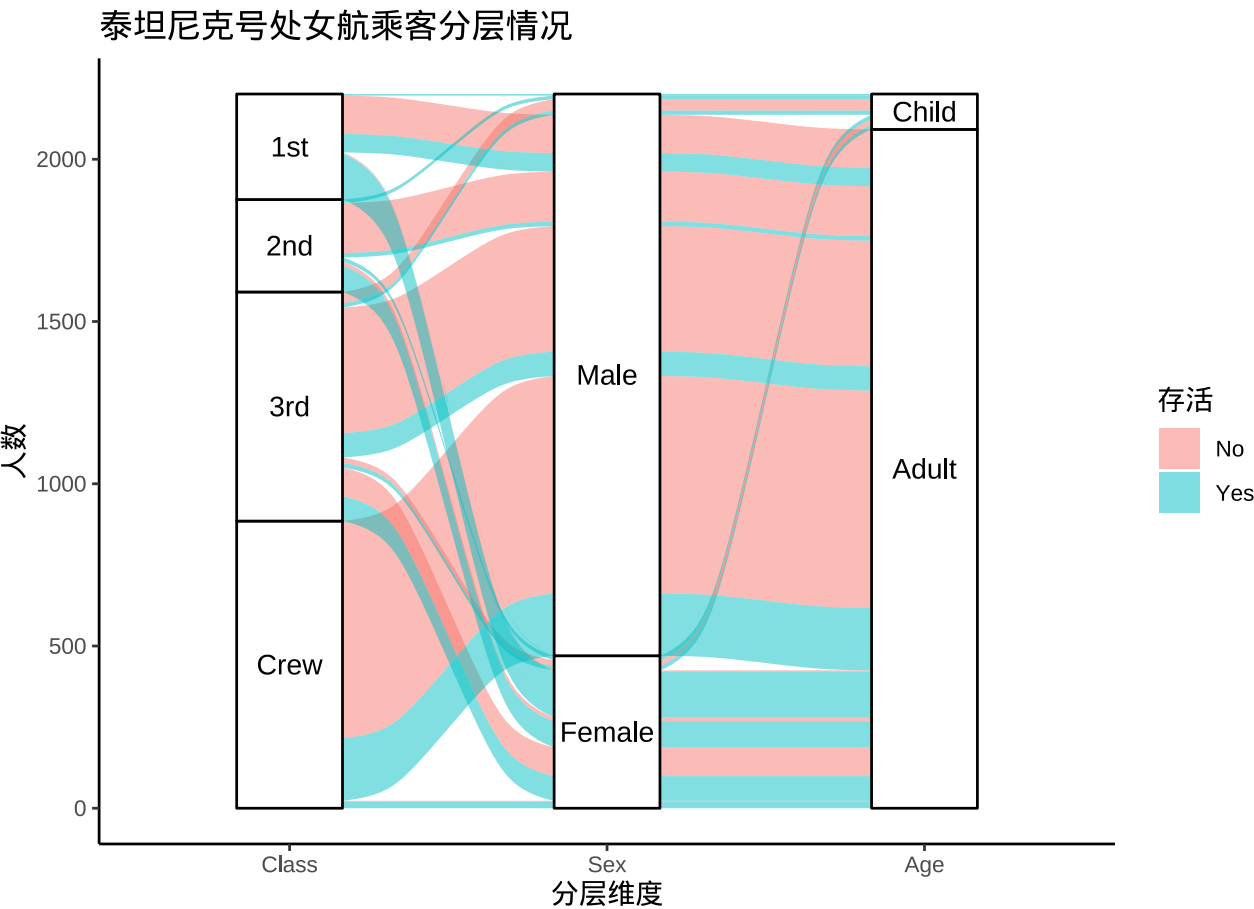
图 16.2: 桑基图展示多维分类数据
