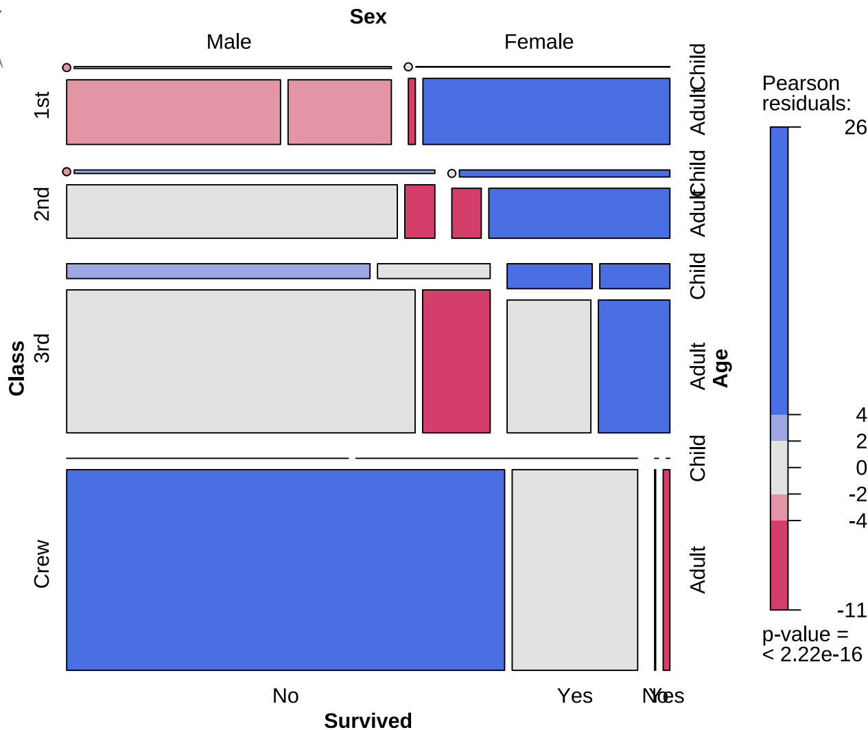
图 16.4: 马赛克图展示多维分类数据
