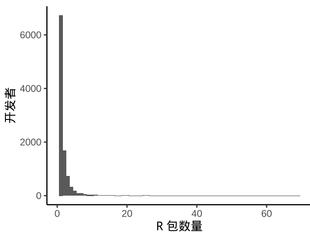
(a) 直方图
