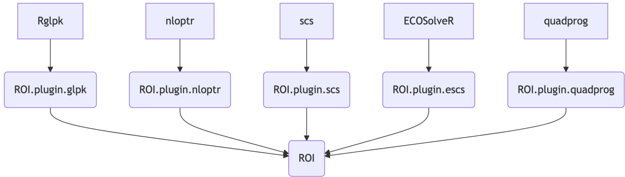
图 23.1: 数值优化扩展包、插件包和 ROI 包的关系图
