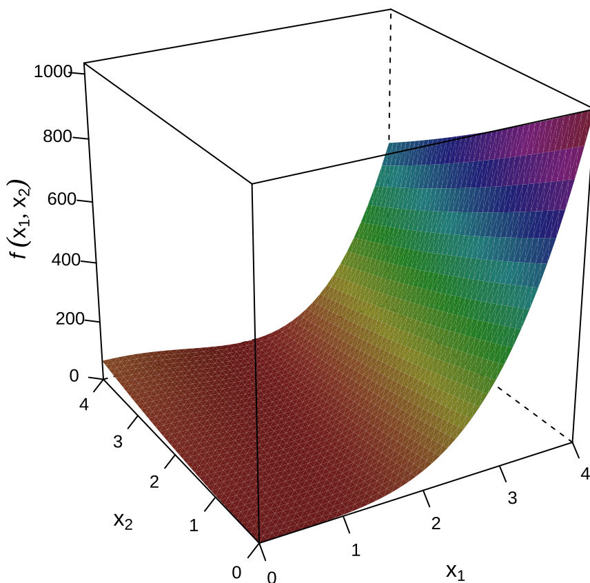
图 23.9: 类香蕉函数的曲面图
