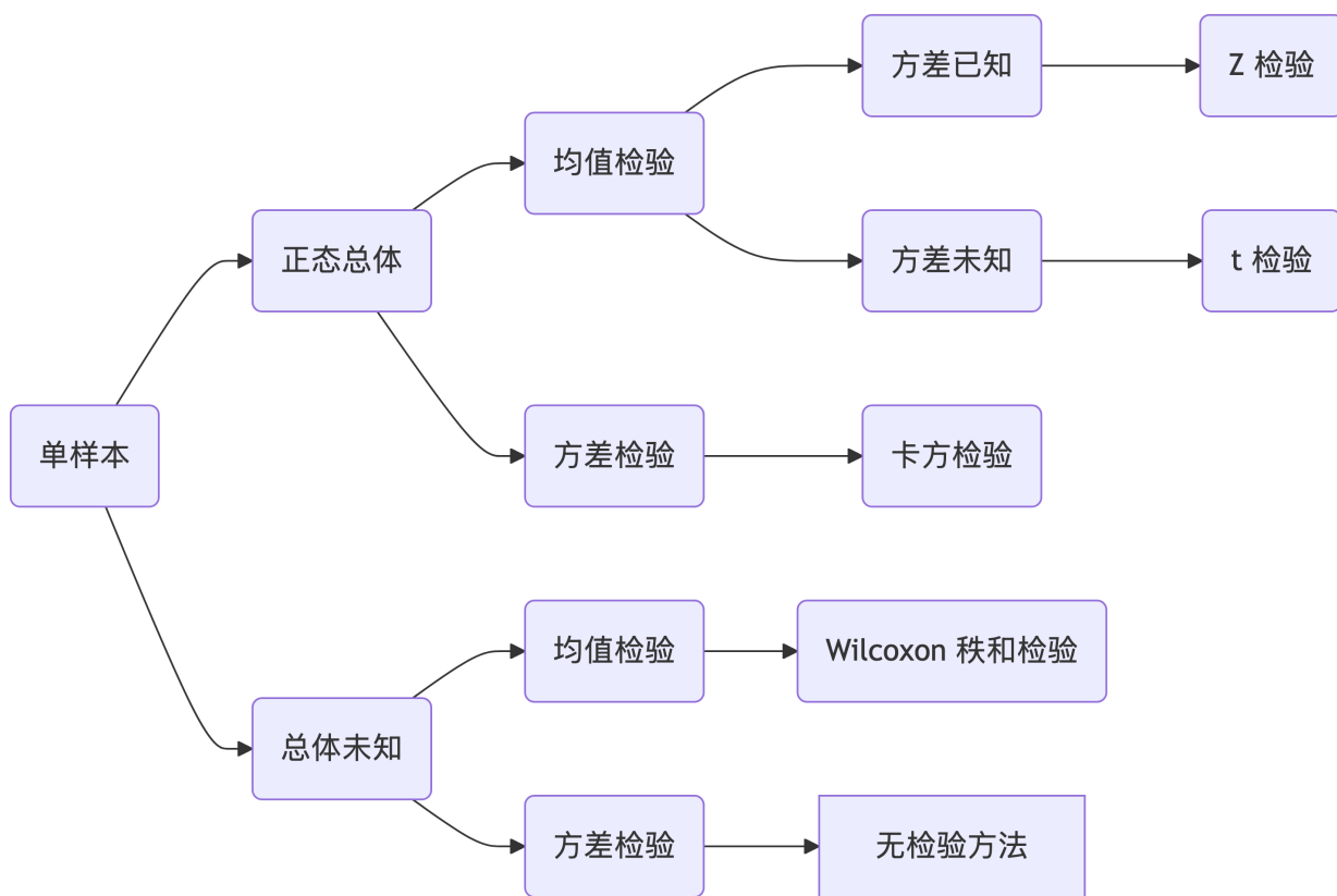
图 14.1: 单样本检验
