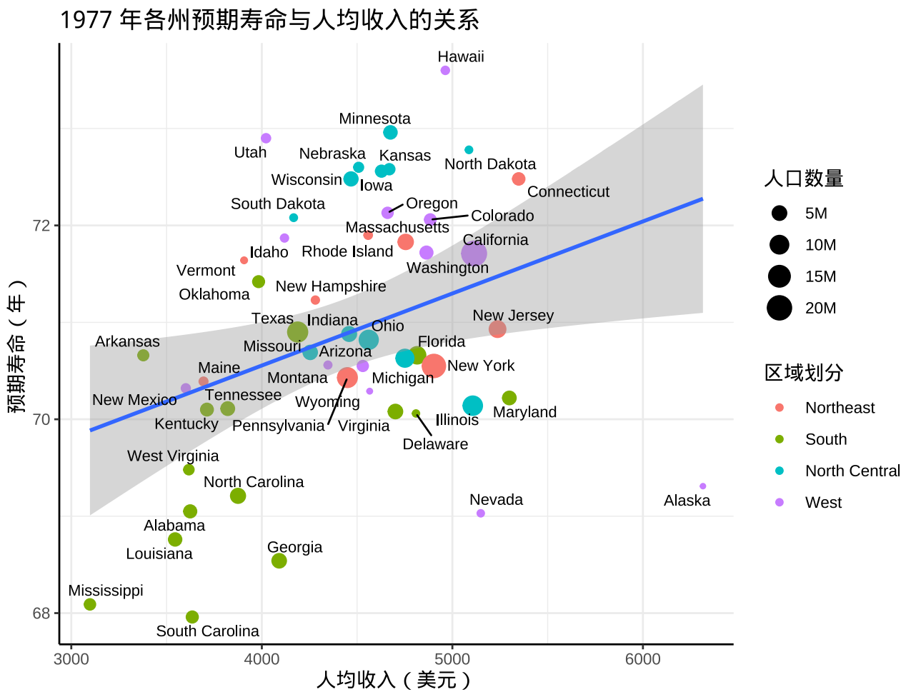
图 15.6: 1977 年美国各州预期寿命与人均收入的关系：回归分析
