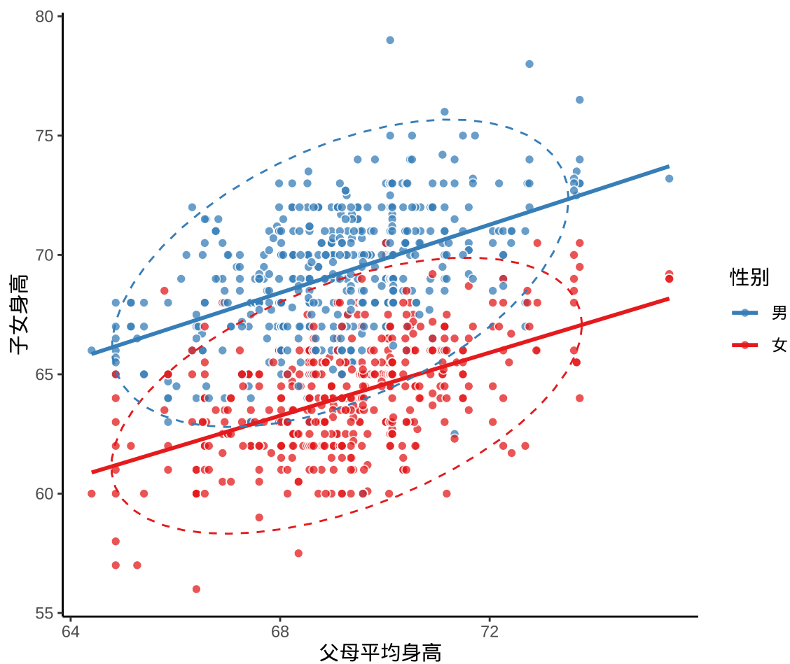
图 15.1: 子代身高与亲代身高的关系
