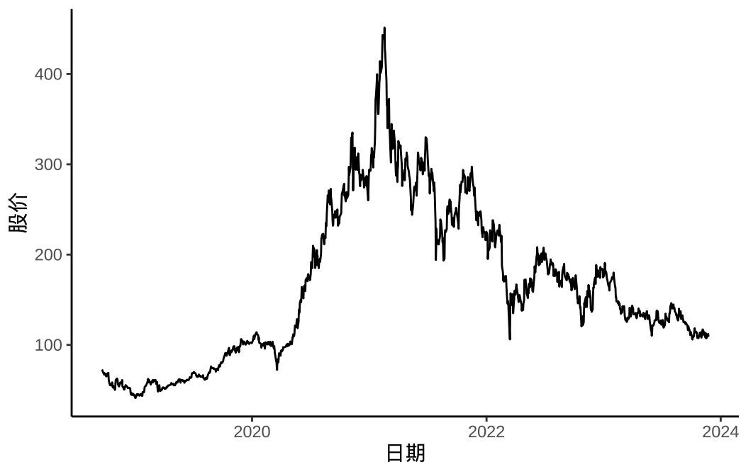
图 21.1: 美团在香港上市以来的股价走势
