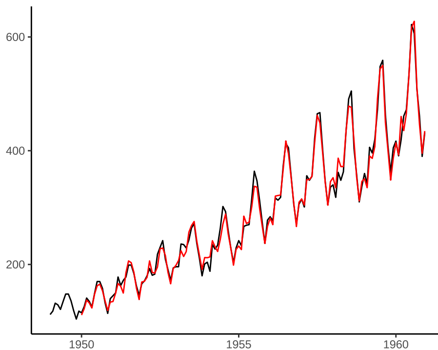
图 21.13: 可乘 Holt-Winters 平滑模型拟合
