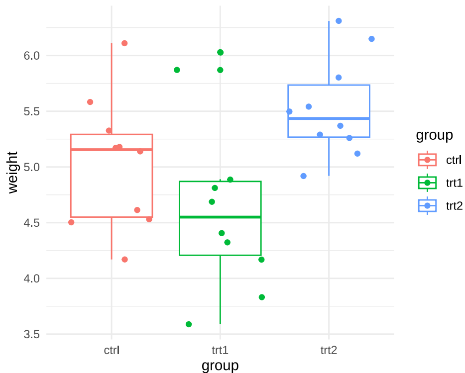
图 14.7: 植物干重
