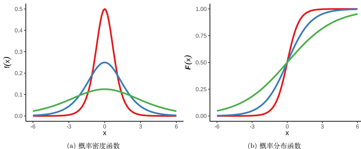
图 22.1: 逻辑斯谛分布
