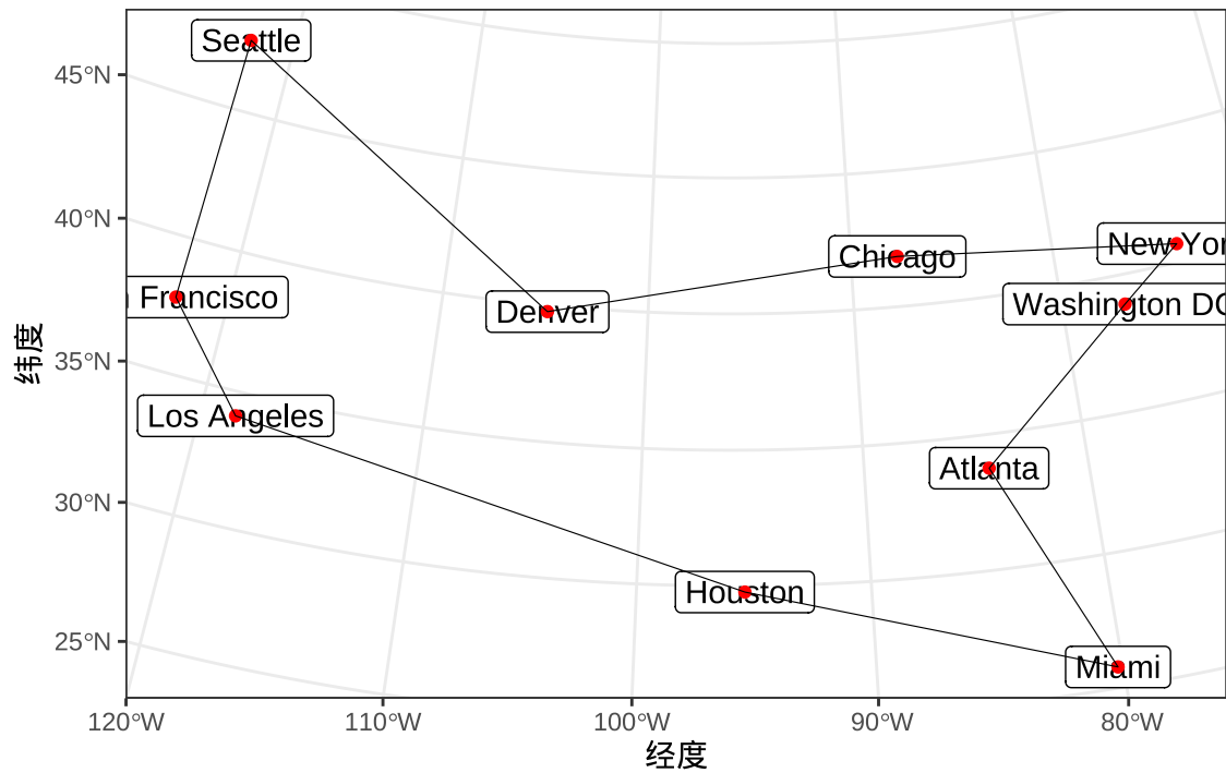
图 24.2: 10 个城市的路线图
