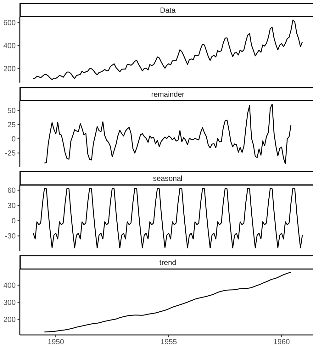
图 21.14: 变化趋势的分解
