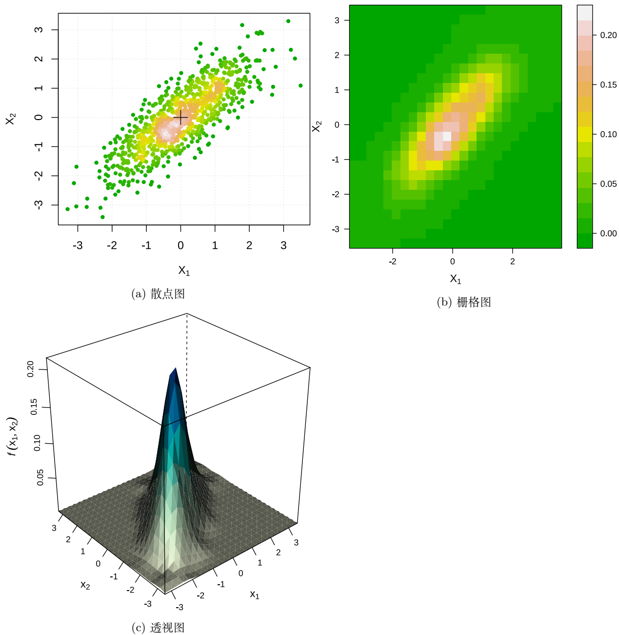
图 13.2: 二维正态分布
