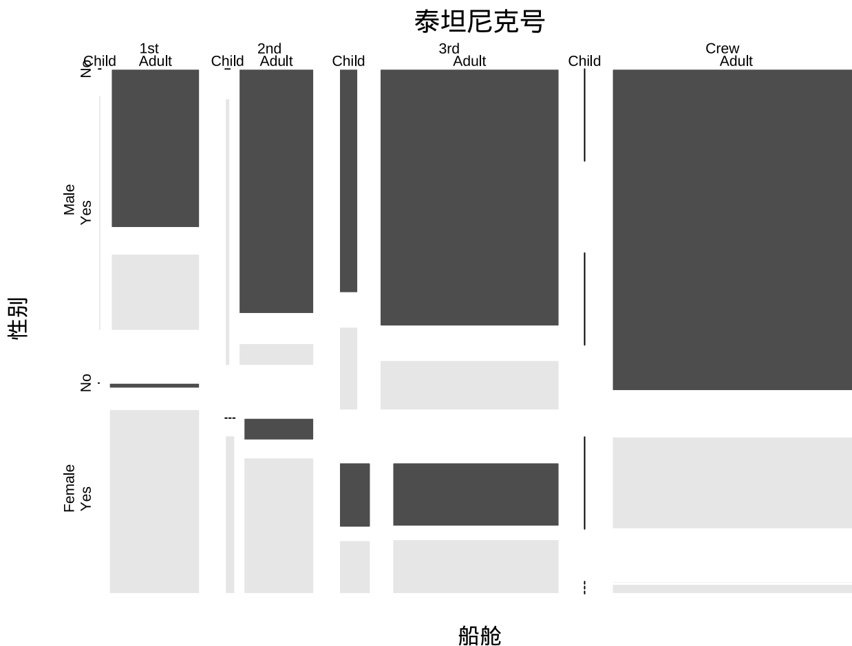
图 16.3: 马赛克图展示多维分类数据
