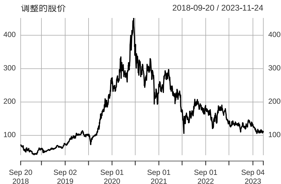
图 21.3: 美团在香港上市以来的股价走势
