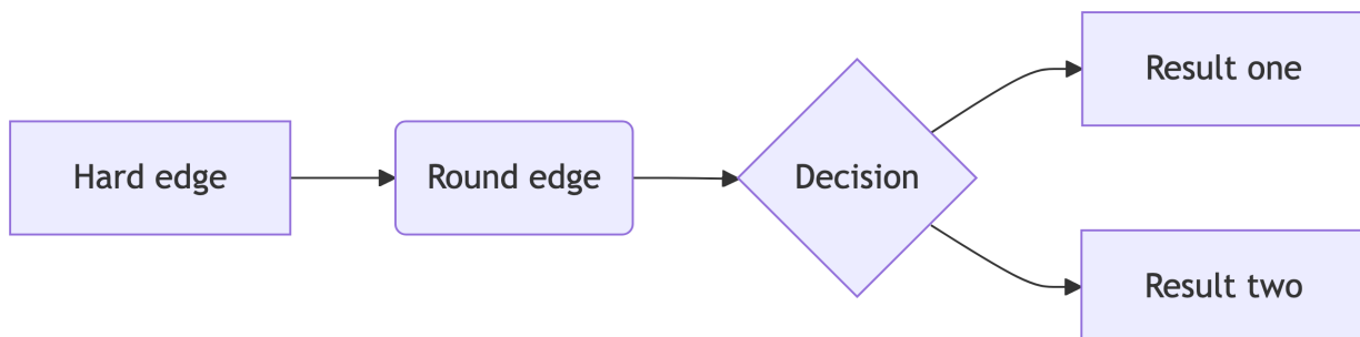
图 10.2: 流程图
