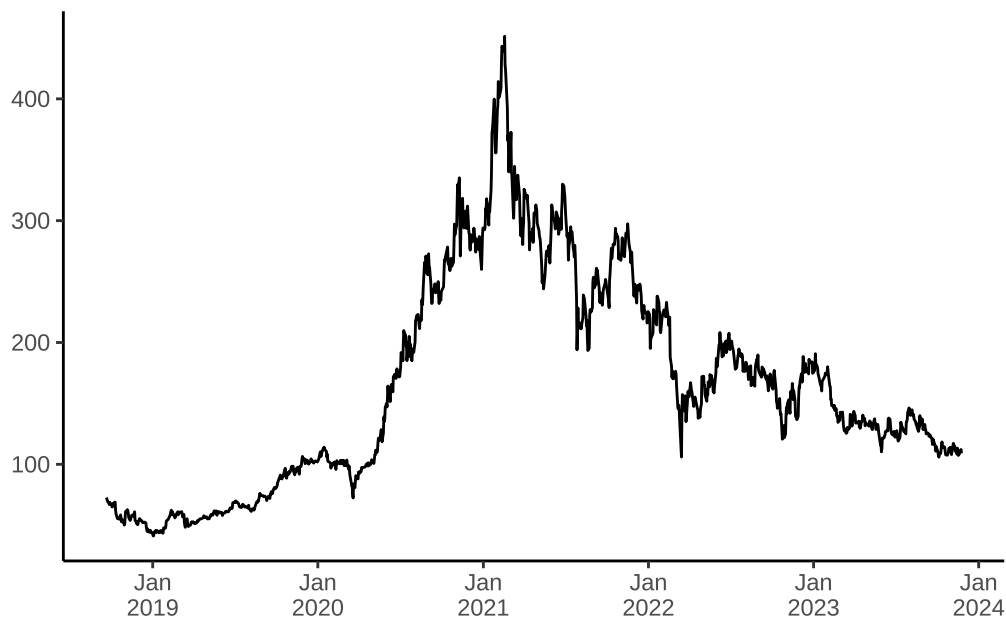
图 21.5: 美团股价走势
