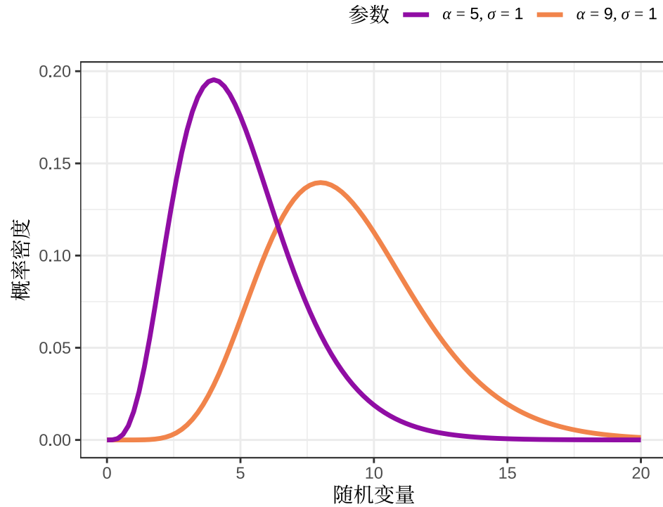
图 24.5: 伽马分布的概率密度函数
