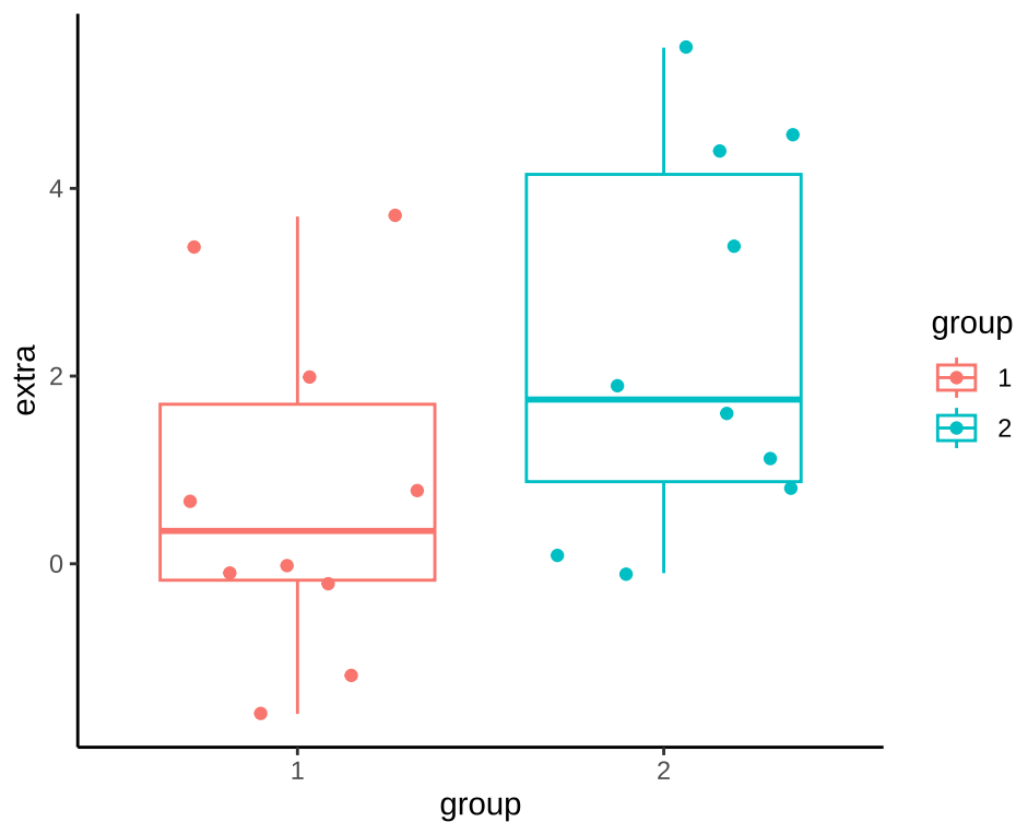
图 14.4: 学生睡眠数据的分布
