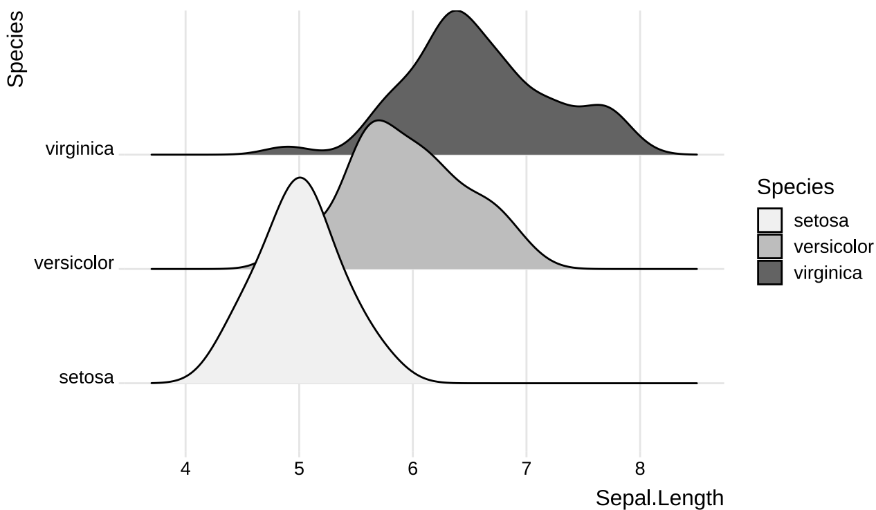
图 14.11: 鸢尾花萼片长度的分布
