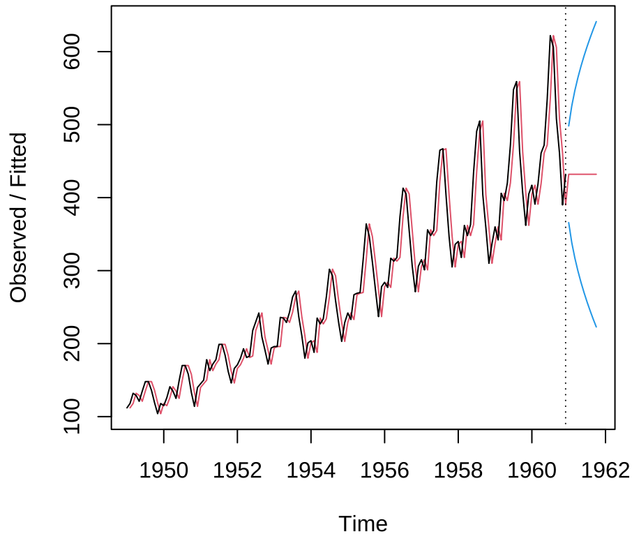
图 21.10: 简单指数平滑模型预测
