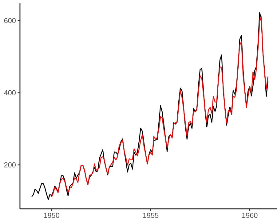
图 21.12: 可加 Holt-Winters 平滑模型拟合
