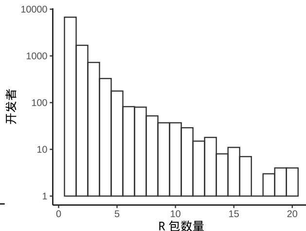
(b) 直方图 (对数尺度)
