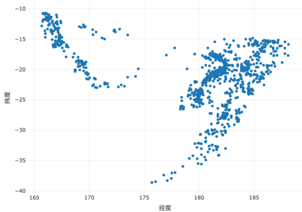
图 6.2: 普通散点图
