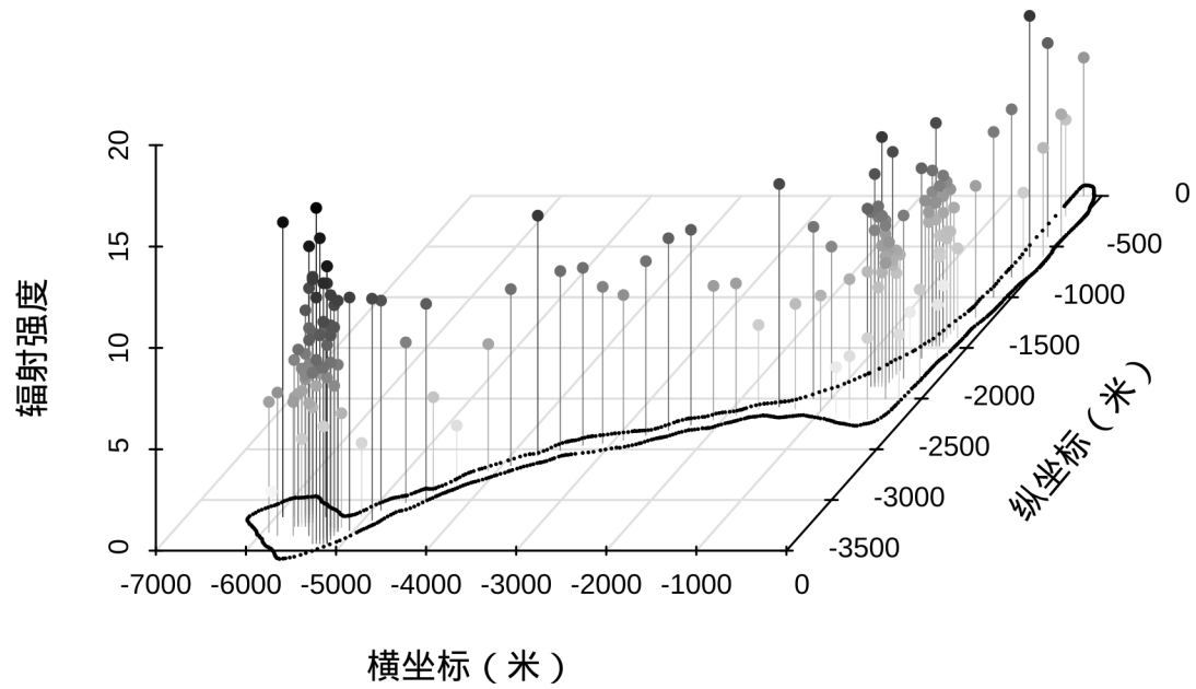
图 19.2: 朗格拉普岛上各采样点的辐射强度
