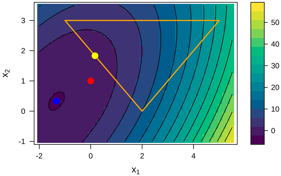
图 23.2: 对比无约束和有约束条件下的解
