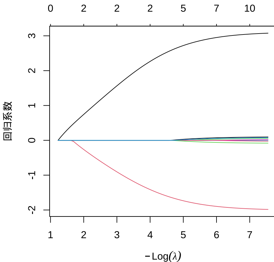
图 22.3: 回归系数的迭代路径
