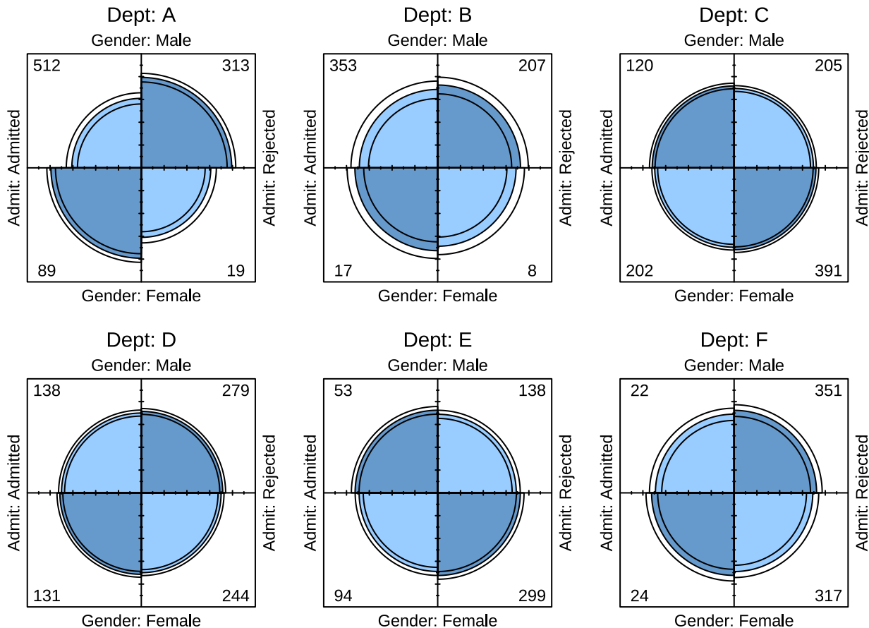
图 16.6: 加州伯克利分校各院系录取情况
