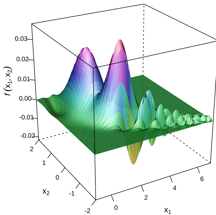
图 23.6: 隐函数图像
