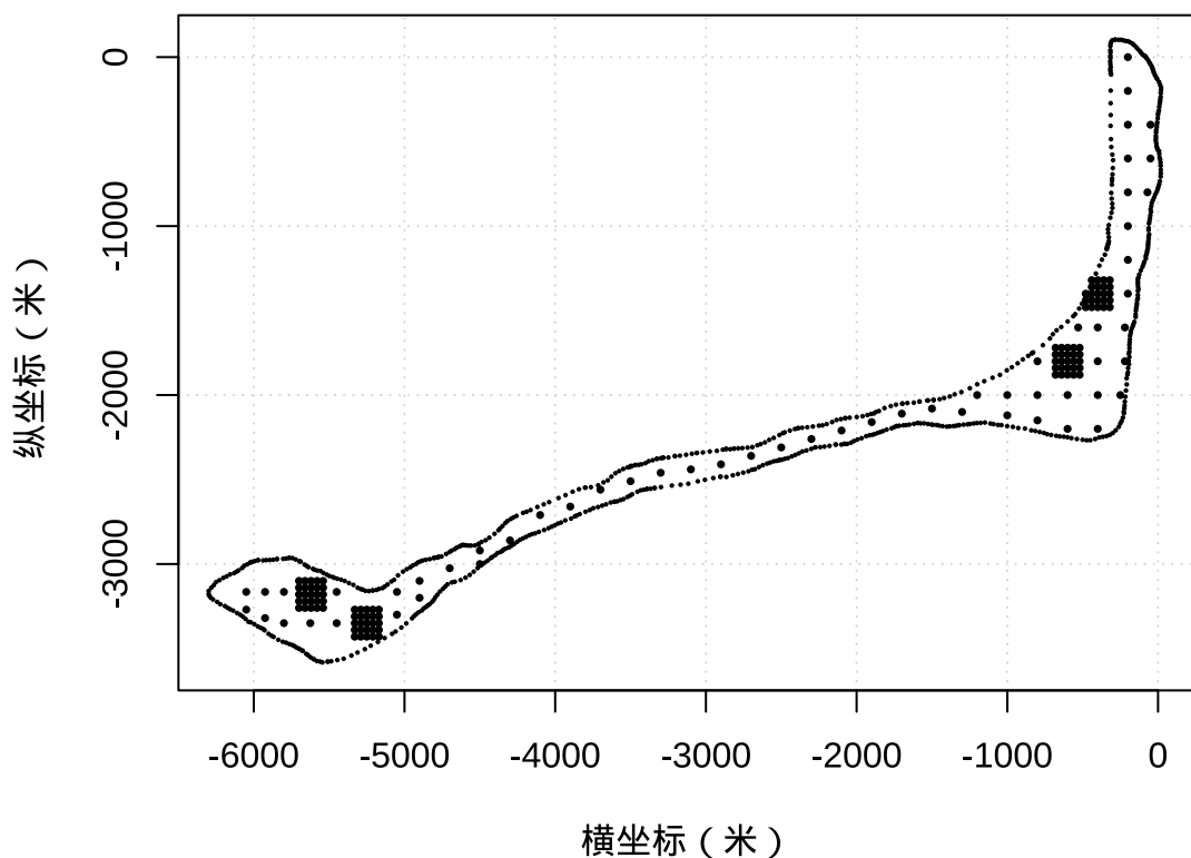
图 19.1: 朗格拉普岛核辐射检测站点及其海岸线
